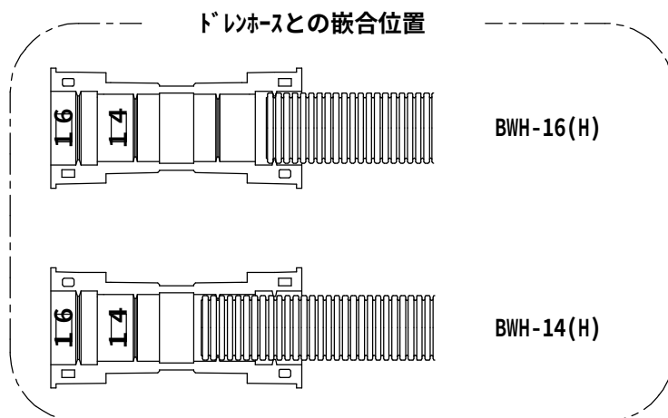
嵌合するドレンパイプ 付属
